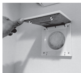
③表面カバーの上のツメ2箇所をアダプターに押し込み固定します
