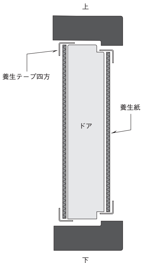
図2 垂直断面図
