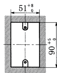
加工穴寸法(単位mm)
