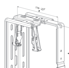
⑧ヘッドレール ブラケット
